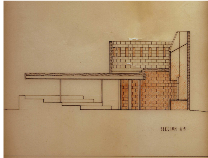
PLANTAS Y SECCIONES
