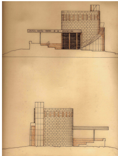
ALZADOS Y SECCIONES
